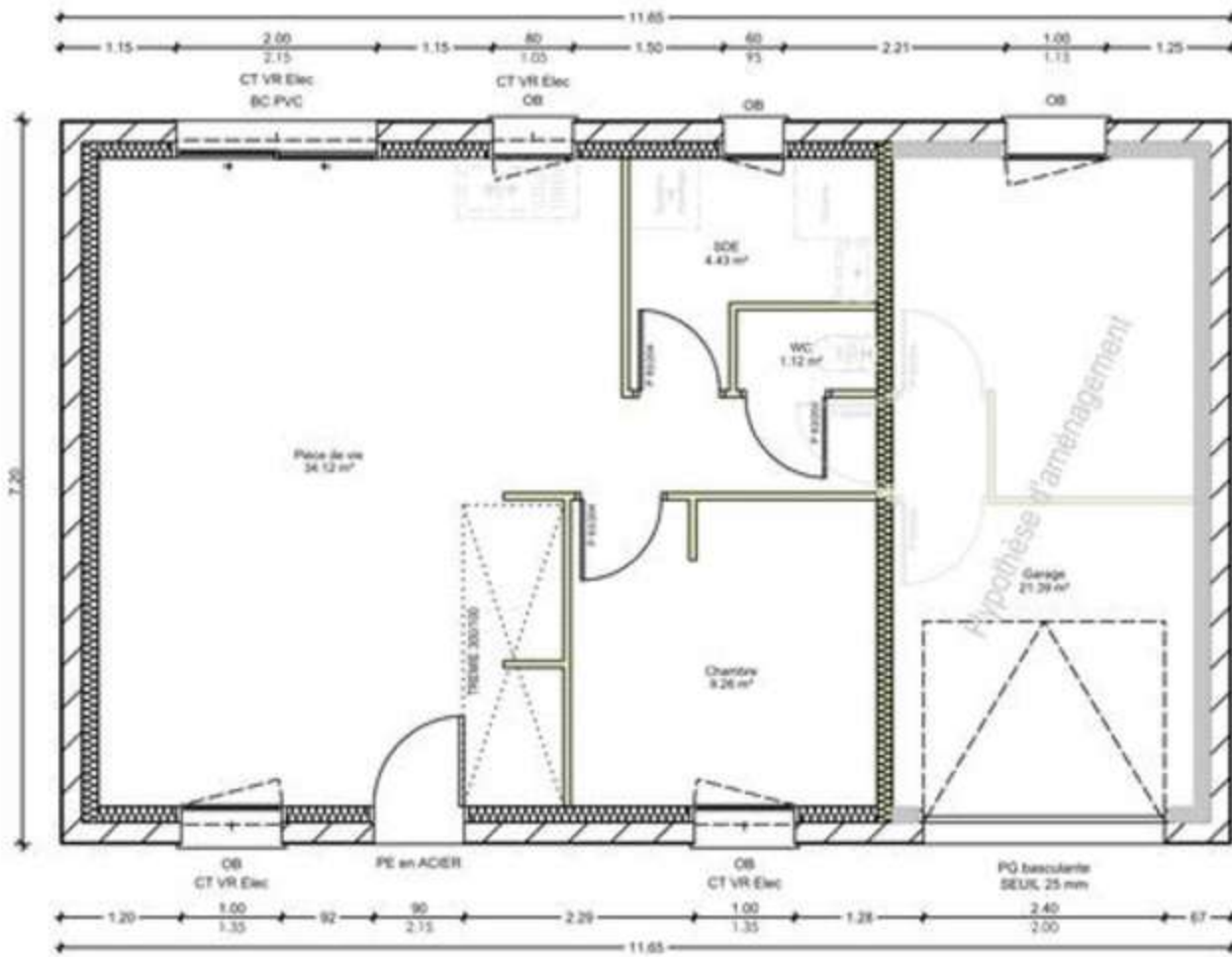
Rez-de-chaussée
