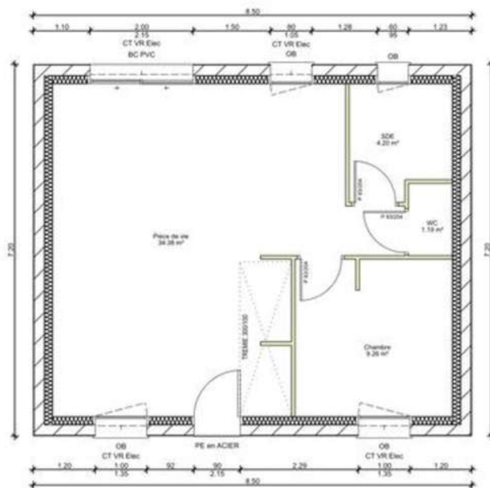
Rez-de-chaussée
